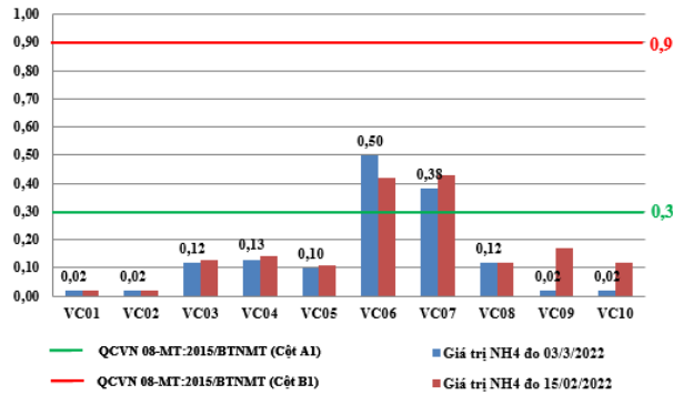
Hình 7: Biểu đồ giá trị \text{NH}_4 tại các vị trí lấy mẫu ngày 03/03/2022
