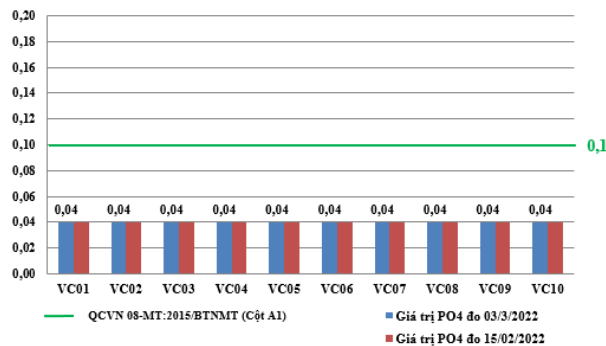
Hình 8: Biểu đồ giá trị \text{PO}_4^{3-} tại các vị trí lấy mẫu ngày 03/03/2022
