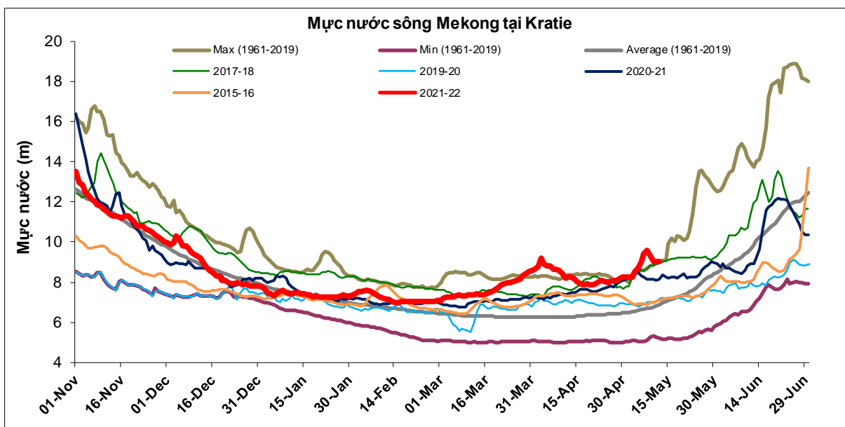
Hình 3. Diễn biến mực nước về qua trạm Kratie, cập nhật ngày 12/5/2022
