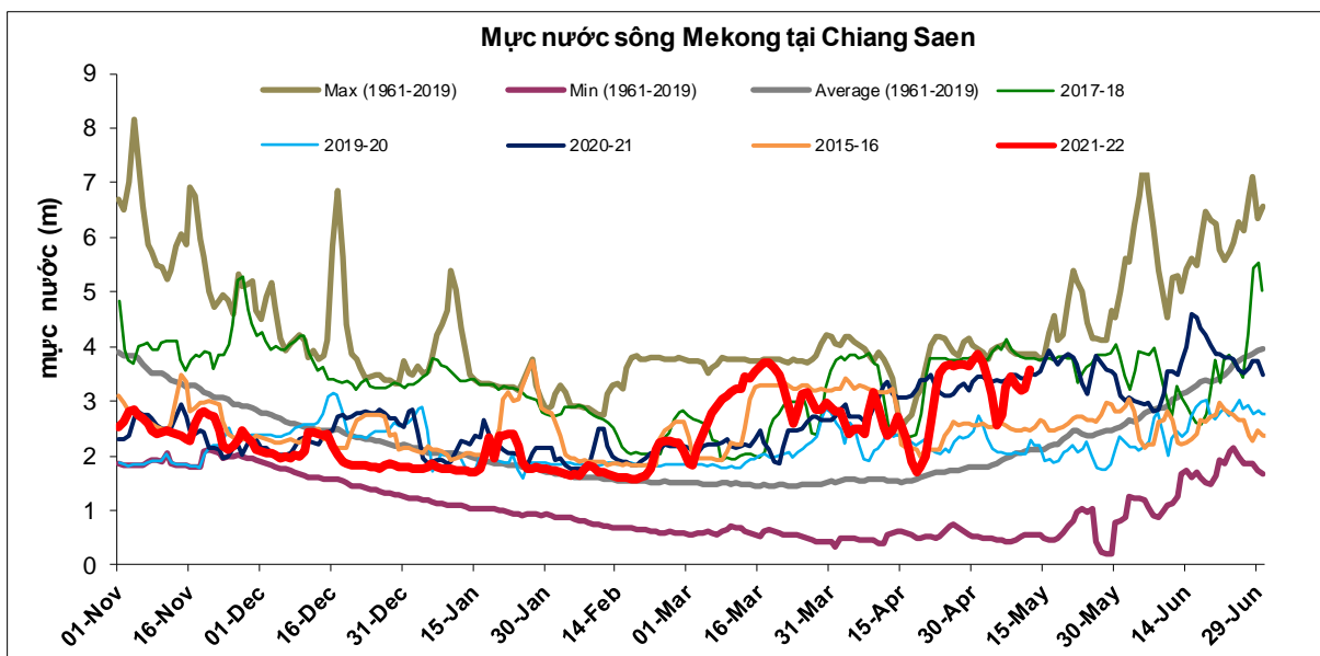
Hình 2. Diễn biến mực nước tại Chiang Saen –Thái Lan, cập nhật 12/5/2022
