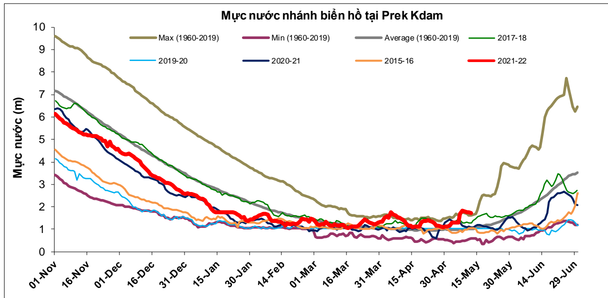
Hình 1. Diễn biến mực nước trạm Prek Kdam - Biển hồ, cập nhật ngày 12/5/2022
