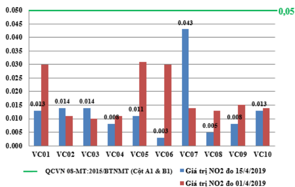
Hình 9: Biểu đồ giá trị \text{NO}_2^- tại các vị trí lấy mẫu ngày 15/4/2019
