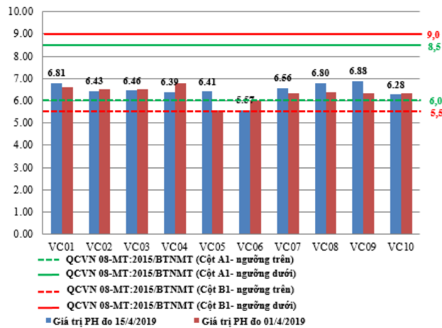
Hình 2: Biểu đồ giá trị pH tại các vị trí lấy mẫu ngày 15/4/2019
