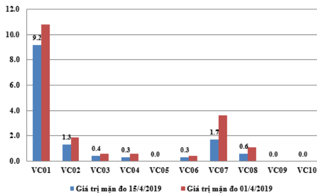
Hình 3: Biểu đồ giá trị mặn tại các vị trí lấy mẫu ngày 15/4/2019
