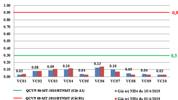
Hình 8: Biểu đồ giá trị \text{NH}_4^+ tại các vị trí lấy mẫu ngày 15/4/2019
