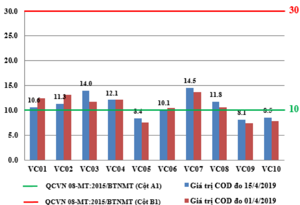
Hình 7: Biểu đồ giá trị COD tại các vị trí lấy mẫu ngày 15/4/2019
