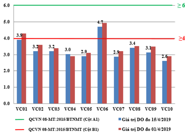
Hình 5: Biểu đồ giá trị DO tại các vị trí lấy mẫu ngày 15/4/2019
