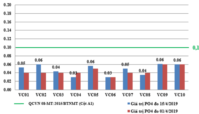
Hình 11: Biểu đồ giá trị PO_4^{3-} tại các vị trí lấy mẫu ngày 15/4/2019
