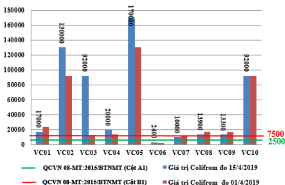
Hình 13: Biểu đồ giá trị Coliform tại các vị trí lấy mẫu ngày 15/4/2019
