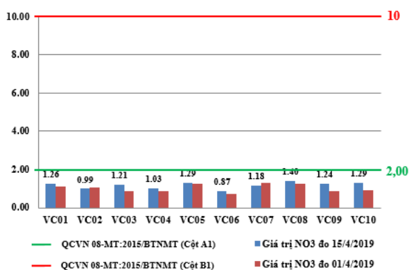
Hình 10: Biểu đồ giá trị \text{NO}_3^- tại các vị trí lấy mẫu ngày 15/4/2019
