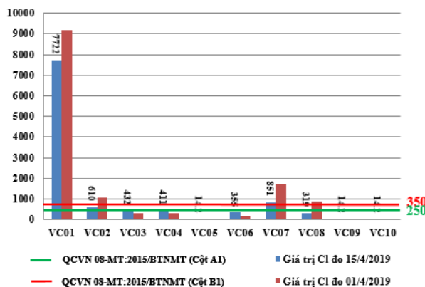
Hình 12: Biểu đồ giá trị Cl^- tại các vị trí lấy mẫu ngày 15/4/2019
