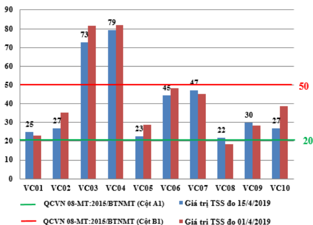
Hình 4: Biểu đồ giá trị TSS tại các vị trí lấy mẫu ngày 15/4/2019
