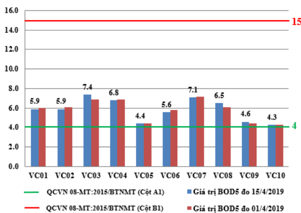
Hình 6: Biểu đồ giá trị BOD 5 tại các vị trí lấy mẫu ngày 15/4/2019
