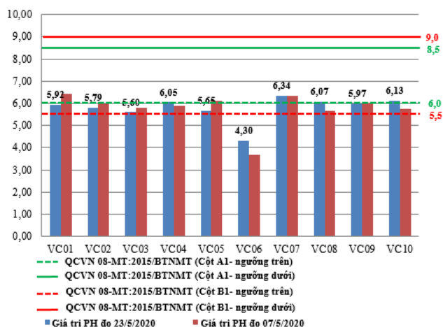
Hình 2: Biểu đồ giá trị pH tại các vị trí lấy mẫu ngày 23/5/2020
