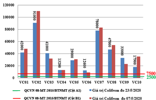
Hình 9: Biểu đồ giá trị Coliform tại các vị trí lấy mẫu ngày 23/5/2020
