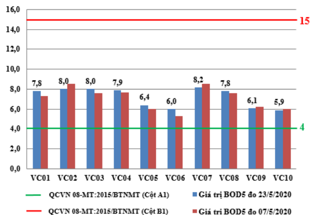
Hình 6: Biểu đồ giá trị BOD 5 tại các vị trí lấy mẫu ngày 23/5/2020
