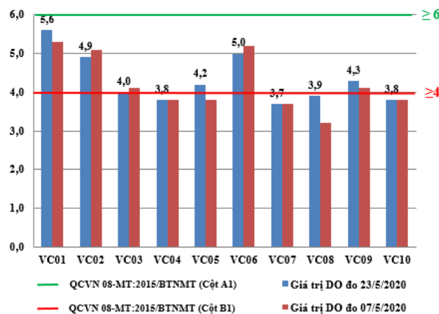
Hình 5: Biểu đồ giá trị DO tại các vị trí lấy mẫu ngày 23/5/2020
