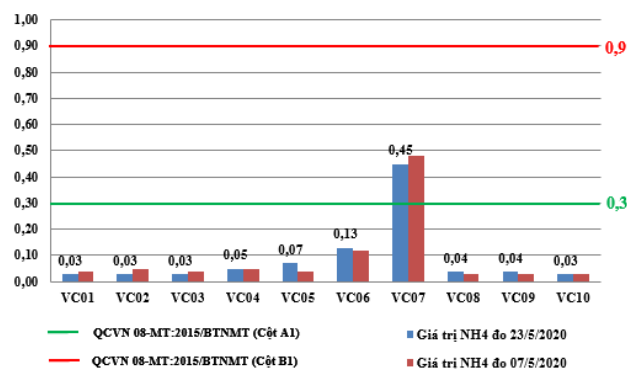
Hình 7: Biểu đồ giá trị NH 4 + tại các vị trí lấy mẫu ngày 23/5/2020
