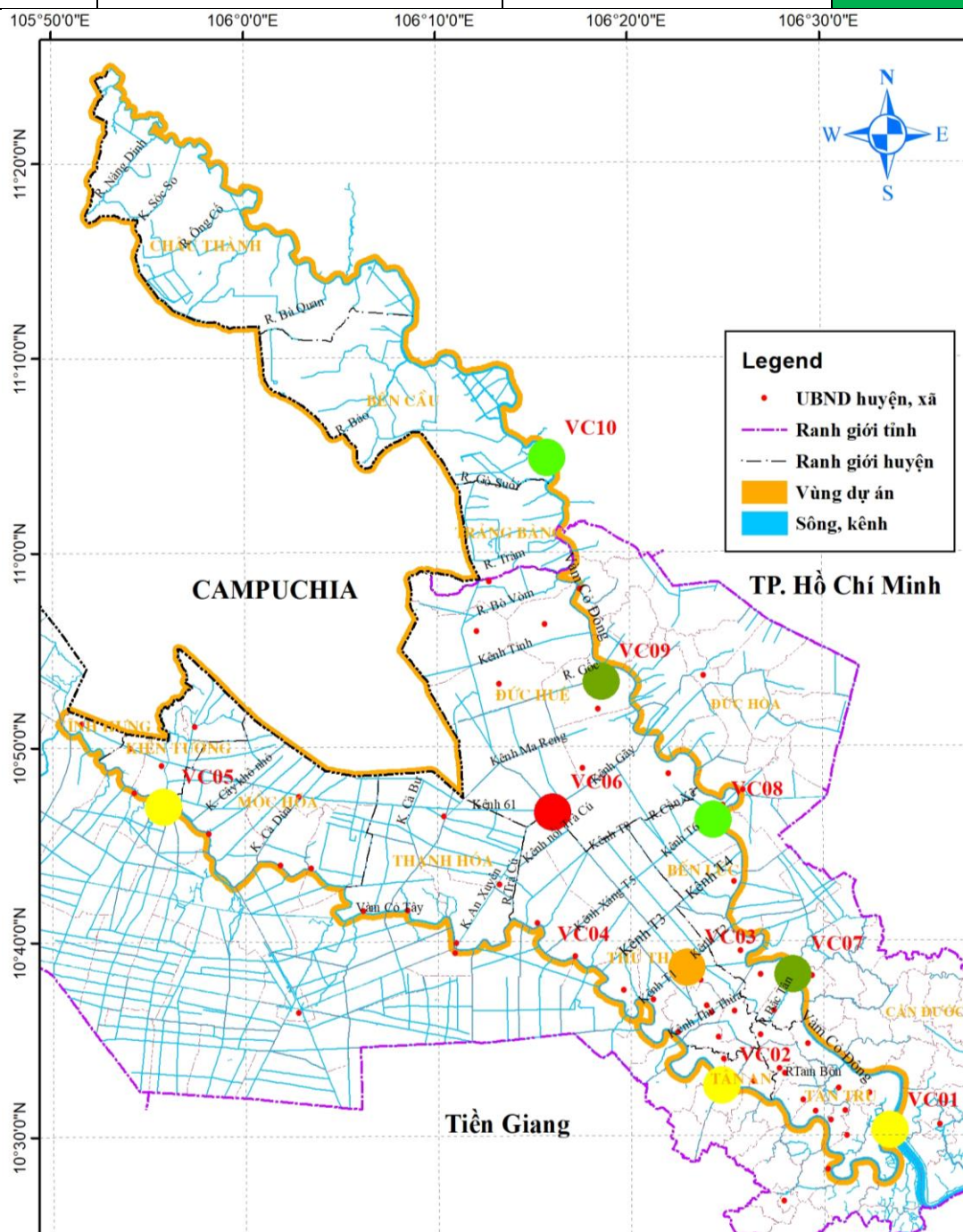
Hình 10: Biểu thị chỉ số WOI tại các vị trí lấy mẫu ngày 23/5/2020
