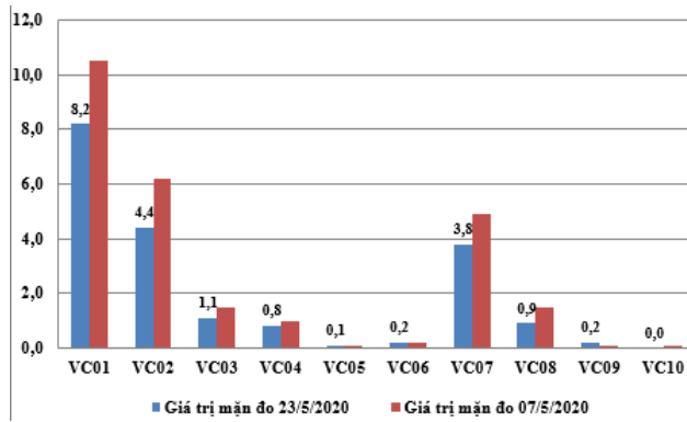
Hình 3: Biểu đồ giá trị độ mặn tại các vị trí lấy mẫu ngày 23/5/2020
