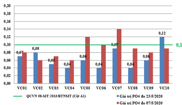
Hình 8: Biểu đồ giá trị PO 4 3- tại các vị trí lấy mẫu ngày 23/5/2020
