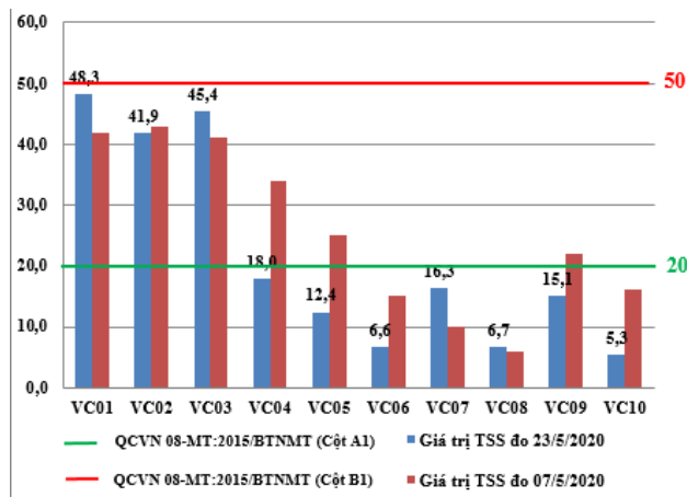
Hình 4: Biểu đồ giá trị TSS tại các vị trí lấy mẫu ngày 23/5/2020
