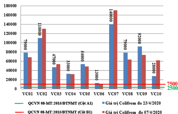
Hình 9: Biểu đồ giá trị Coliform tại các vị trí lấy mẫu ngày 23/4/2020
