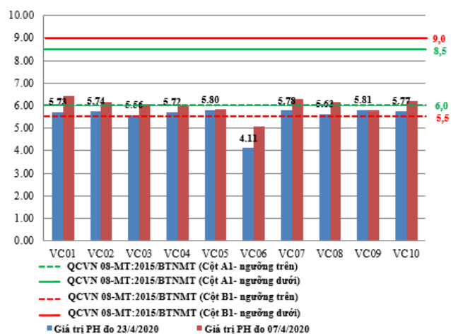
Hình 2: Biểu đồ giá trị pH tại các vị trí lấy mẫu ngày 23/4/2020
