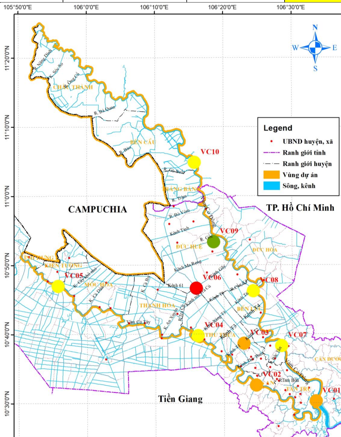
Hình 10: Biểu thị chỉ số WQI tại các vị trí lấy mẫu ngày 23/4/2020
