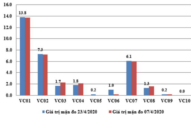
Hình 3: Biểu đồ giá trị mặn tại các vị trí lấy mẫu ngày 23/4/2020
