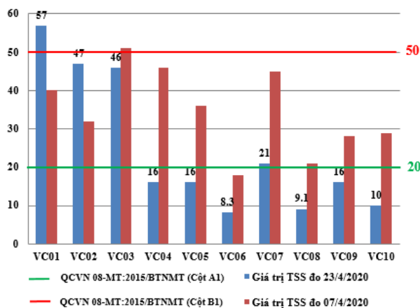
Hình 4: Biểu đồ giá trị TSS tại các vị trí lấy mẫu ngày 23/4/2020
