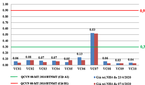
Hình 7: Biểu đồ giá trị NH 4 + tại các vị trí lấy mẫu ngày 23/4/2020
