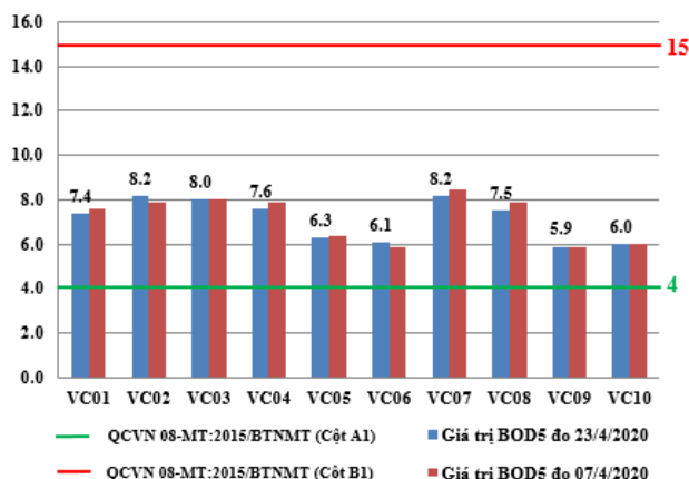
Hình 6: Biểu đồ giá trị BOD 5 tại các vị trí lấy mẫu ngày 23/4/2020
