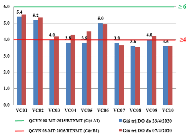
Hình 5: Biểu đồ giá trị DO tại các vị trí lấy mẫu ngày 23/4/2020
