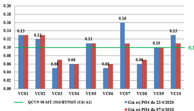
Hình 8: Biểu đồ giá trị PO 4 3- tại các vị trí lấy mẫu ngày 23/4/2020
