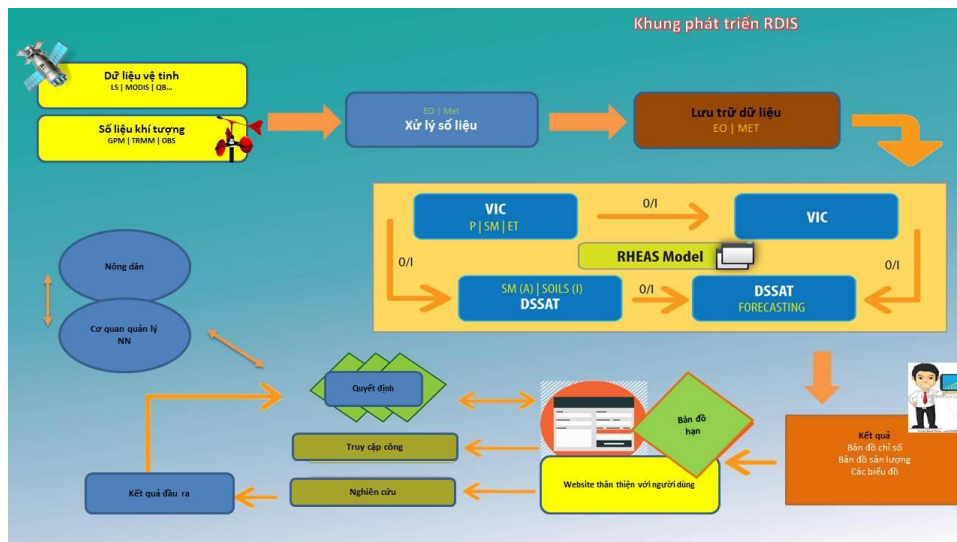
Hình 5. Chu trình dự báo hạn hán bằng phần mềm RHEAS (ADPC)
