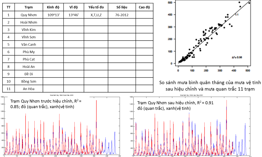
Hình 4. Kiểm định mưa vệ tinh theo mưa trạm mặt đất
