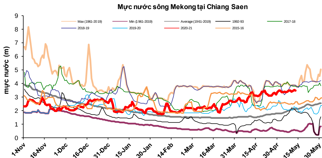
Hình 2. Diễn biến mực nước (cao độ tương đối) tại Chiang Saen –Thái Lan, cập nhật 13/05/2021
