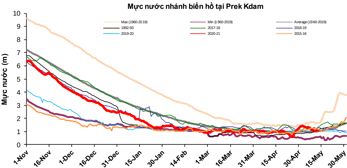
Hình 1. Diễn biến nước trạm Prek Kdam - Biển hồ, cập nhật ngày 13/05/2021
