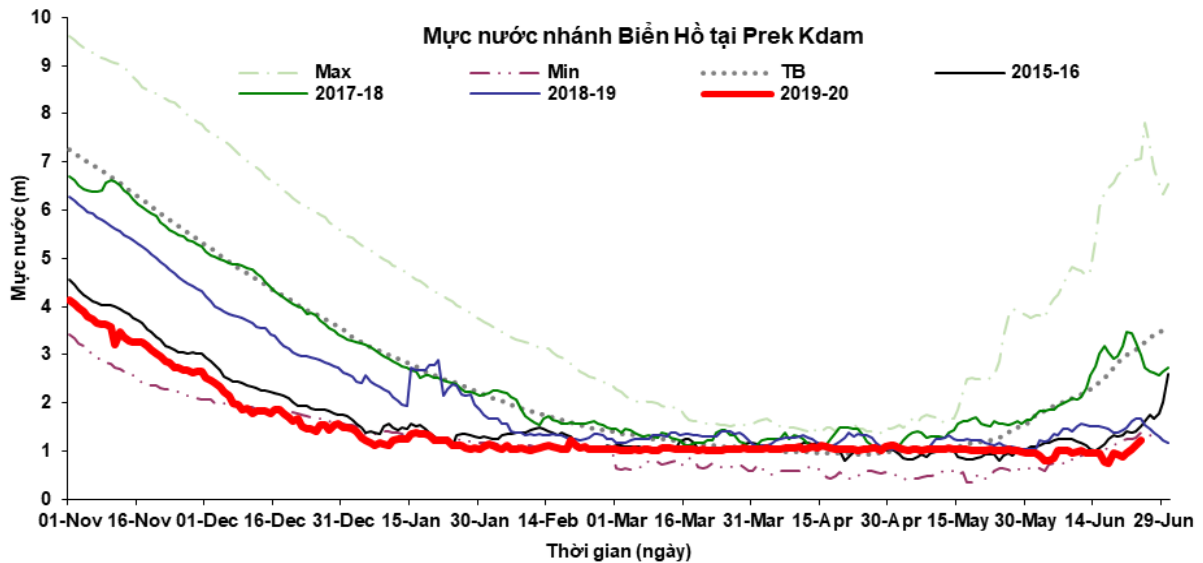
Hình 1. Diễn biến nước trạm Prek Kdam - Biển hồ, cập nhật ngày 24/6
