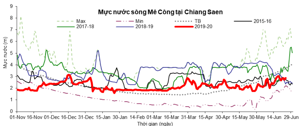
Hình 2. Diễn biến mực nước (cao độ tương đối) tại Chiang Saen –Thái Lan, cập nhật 24/6/2020
