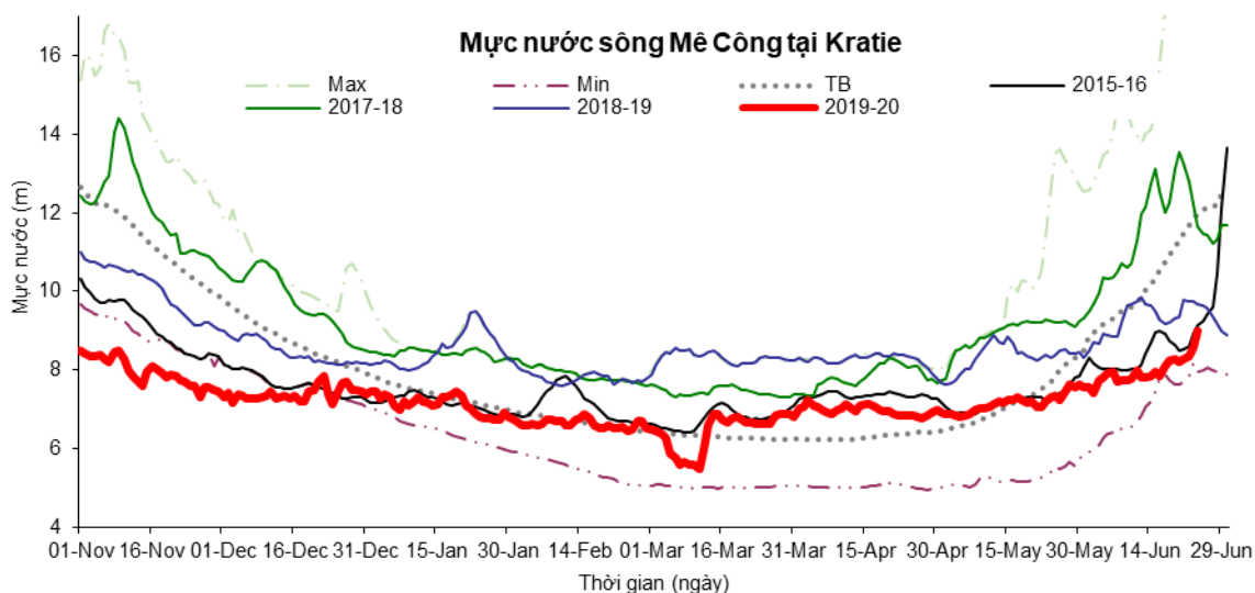
Hình 3. Diễn biến mực nước về qua trạm Kratie, cập nhật ngày 24/6/2020
