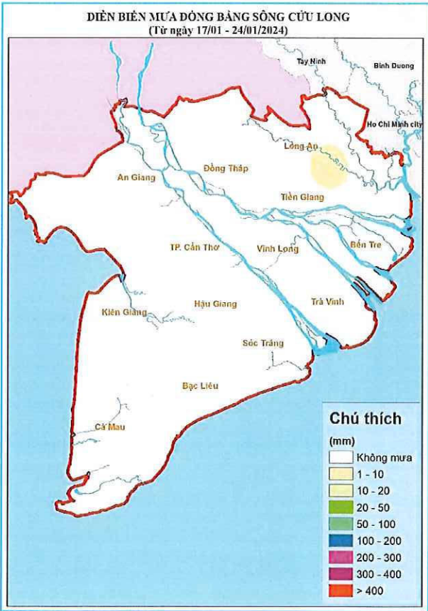
Hình 4. Bản đồ lũy tích lượng mưa trên vùng ĐBSCL (từ ngày 17/01 đến 24/01/2024)
