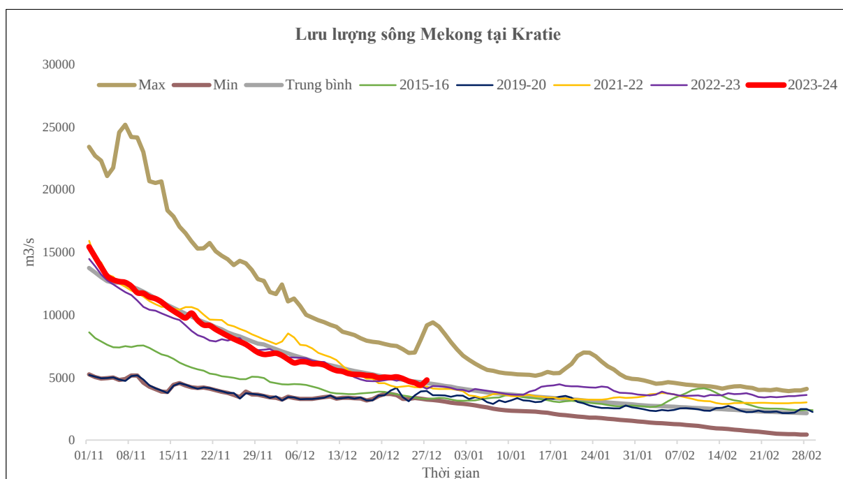
Hình 1. Diễn biến lưu lượng tại Kratie đến tháng 12 năm 2023 và một số năm cùng kỳ
