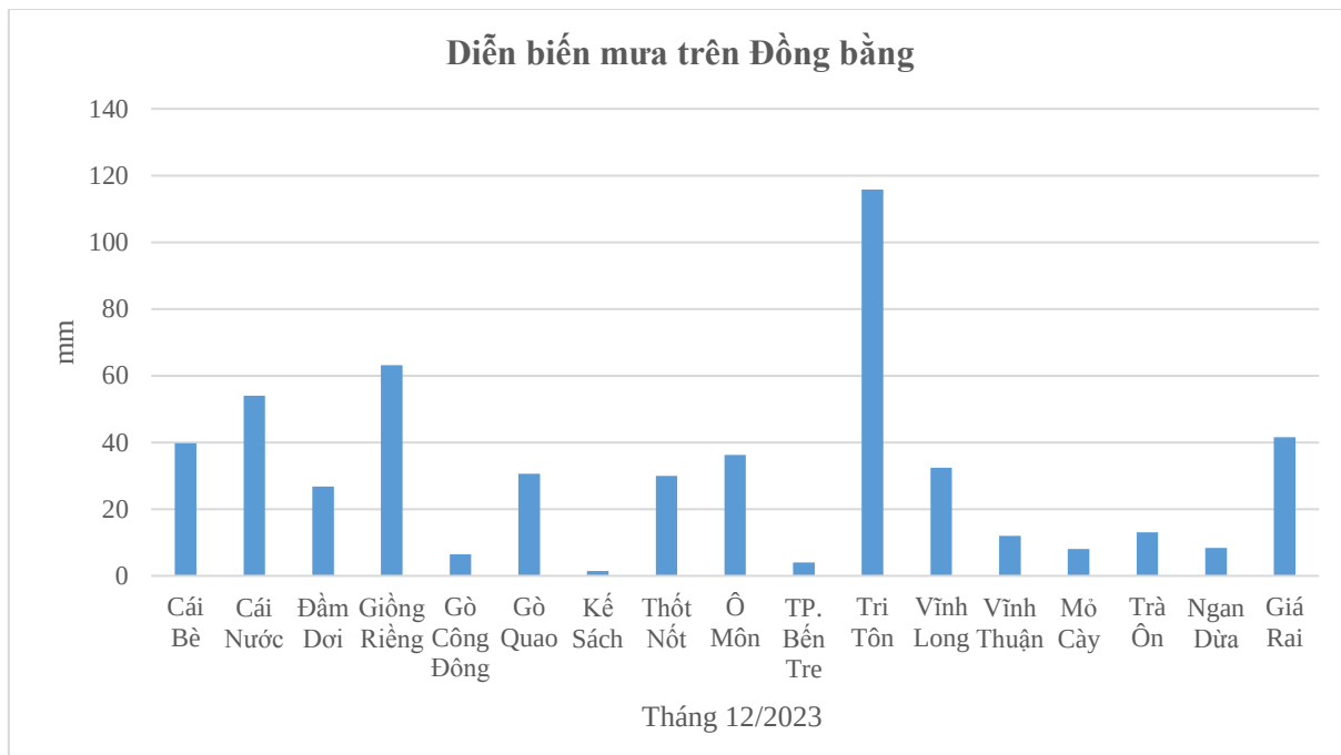
Hình 2: Diễn biến mưa trên đồng bằng sông Cửu Long trong tháng 12/2023
