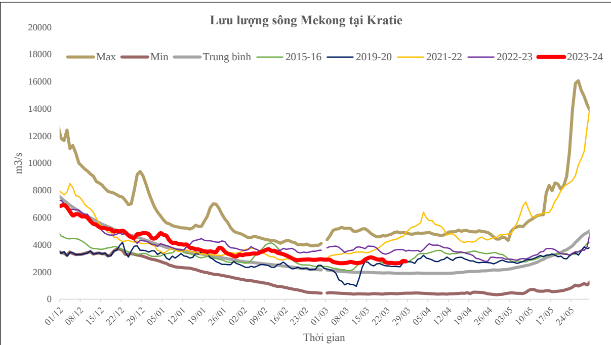
Hình 1. Diễn biến lưu lượng tại Kratie đến tháng 03 năm 2024 và một số năm cùng kỳ
