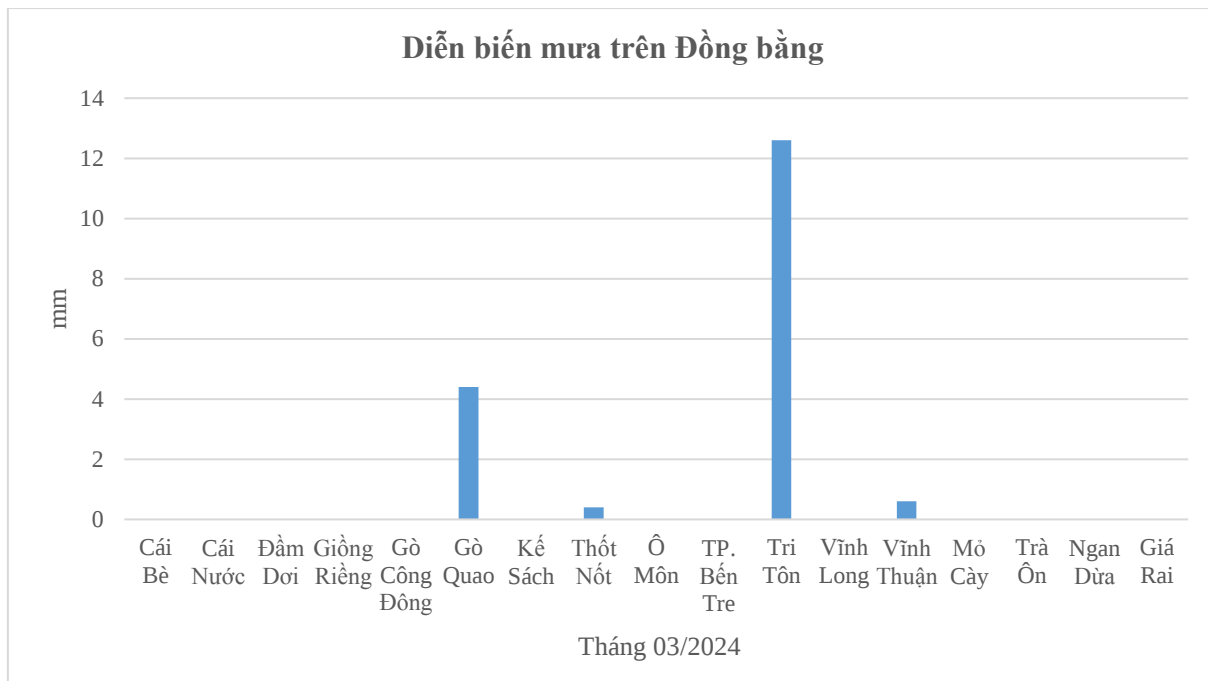
Hình 2: Diễn biến mưa trên đồng bằng sông Cửu Long trong tháng 03/2024
