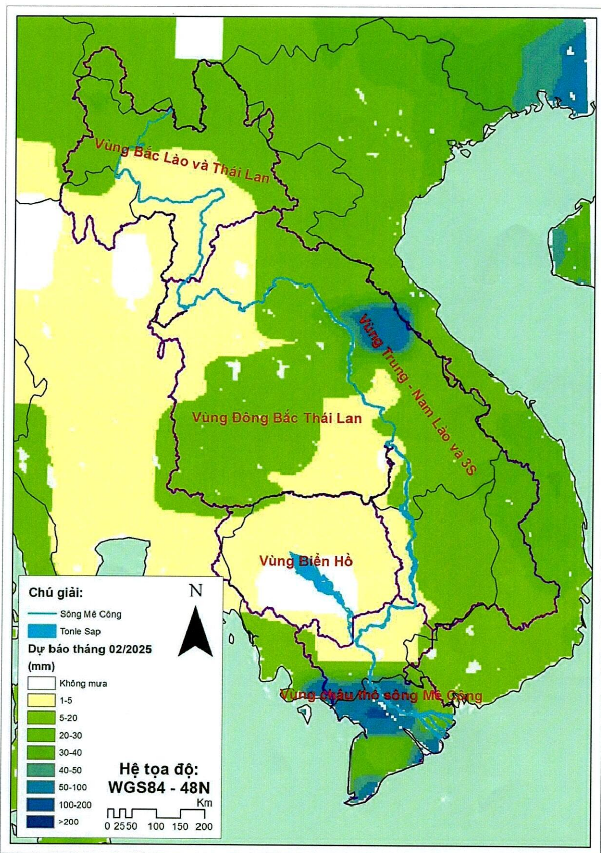
Bản đồ 01: Phân bố mưa trên Hạ lưu vực Mê Công tháng 02/2025
