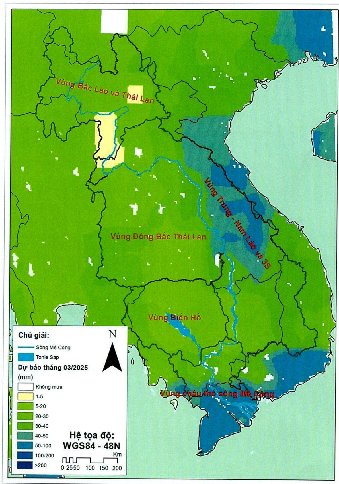
Bản đồ 02: Dự báo mưa trên Hạ lưu vực Mê Công từ tháng 03/2025
