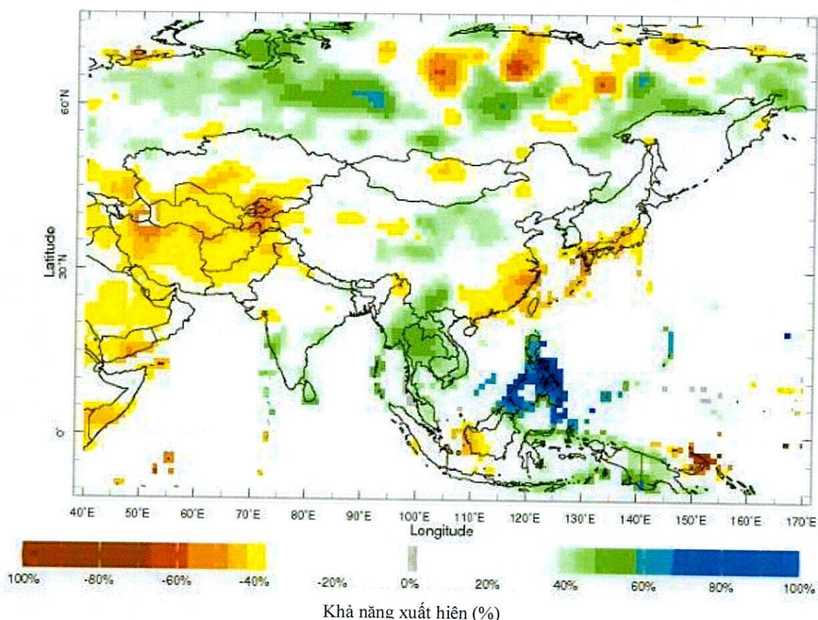
Hình 2.2: Dự báo khả năng xuất hiện mưa mùa kiệt tháng 03/2025 trên lưu vực Mê Công
