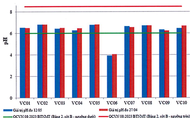
Hình 2: Biểu đồ giá trị pH tại các vị trí lấy mẫu ngày 11-13/05
