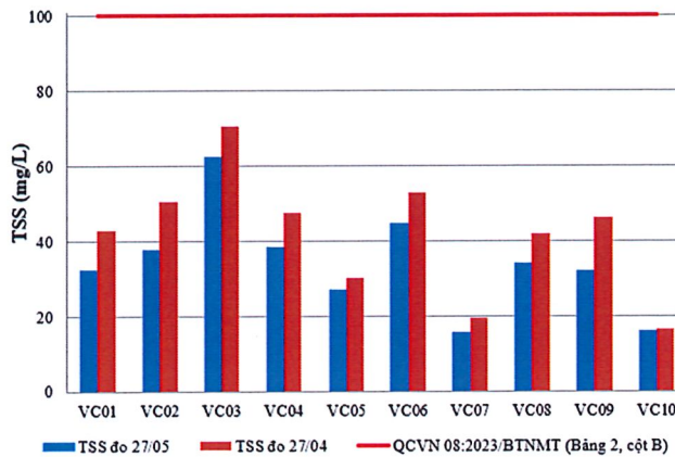
Hình 4: Biểu đồ giá trị TSS tại các vị trí lấy mẫu ngày 11-13/05
