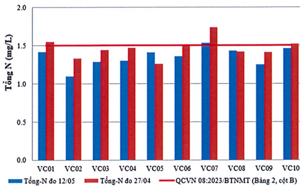
Hình 7: Biểu đồ giá trị tổng N tại các vị trí lấy mẫu ngày 11-13/05
