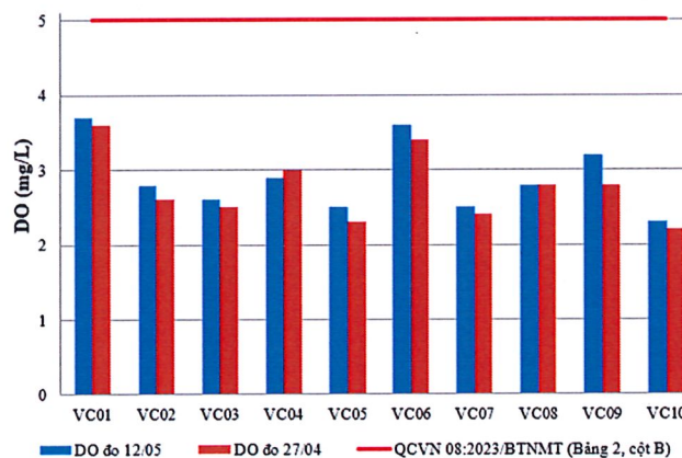
Hình 5: Biểu đồ giá trị DO tại các vị trí lấy mẫu ngày 11-13/05
