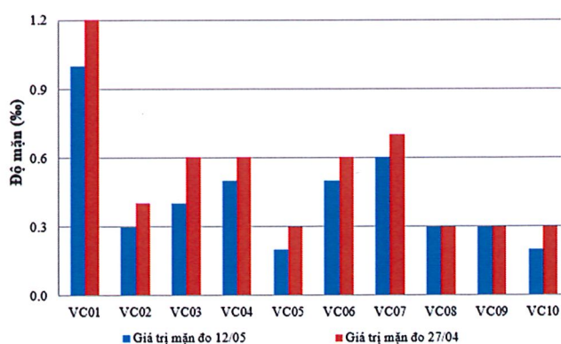
Hình 3: Biểu đồ giá trị mặn tại các vị trí lấy mẫu ngày 11-13/05
