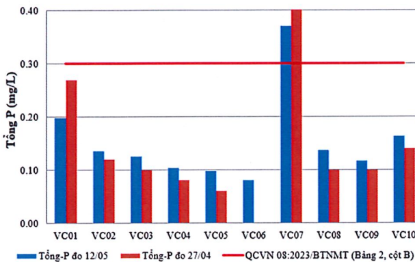
Hình 8: Biểu đồ giá trị tổng P tại các vị trí lấy mẫu ngày 11-13/05
