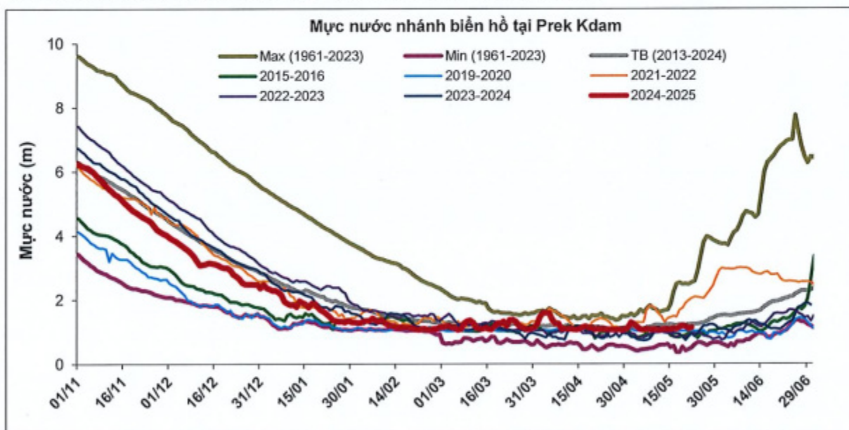
Hình 1. Diễn biến mực nước trạm Prek Kdam - Biển hồ, cập nhật ngày 22/5/2025
