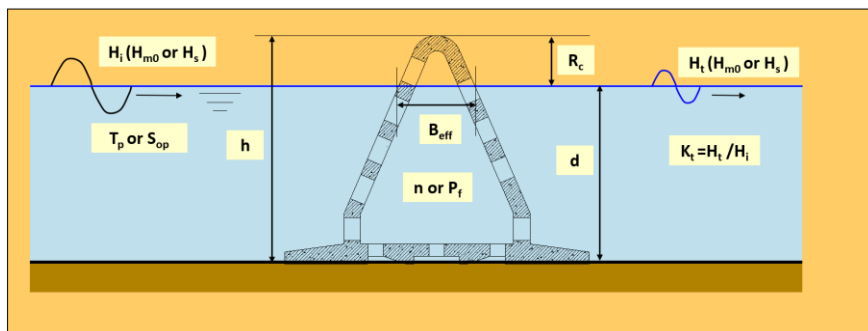
Hình 1-2. Các thông số cơ bản ảnh hưởng đến hệ số truyền sóng K_t
