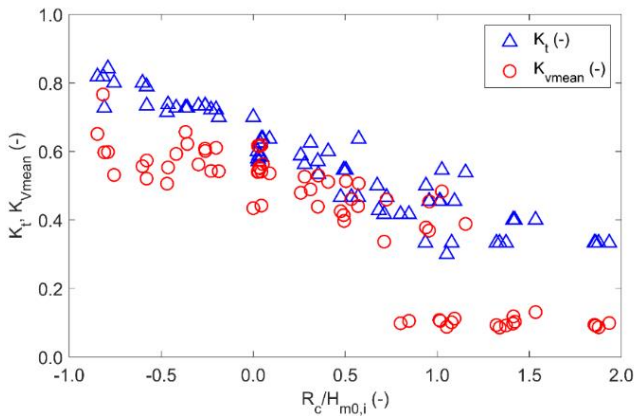
Hình 3-13. Quan hệ hệ số K_t , K_{Vmean} và chiều cao lưu không R_c .
