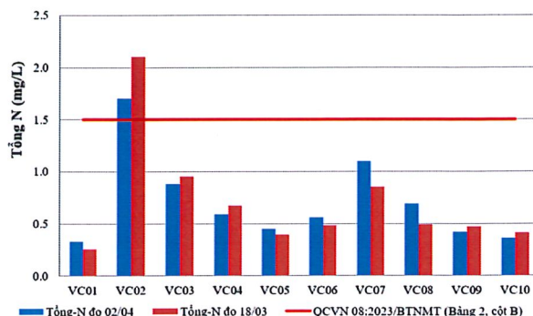
Hình 7: Biểu đồ giá trị tổng N tại các vị trí lấy mẫu ngày 01-03/04
