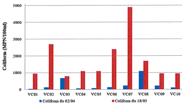
Hình 9: Biểu đồ giá trị Coliform tại các vị trí lấy mẫu ngày 01-03/04
