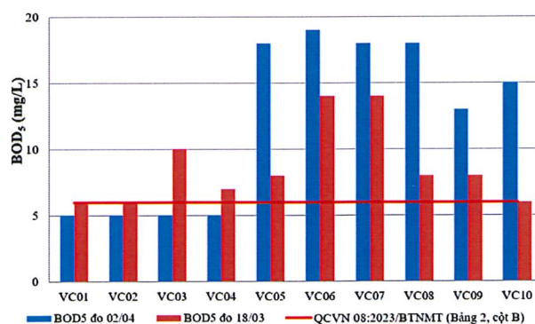
Hình 6: Biểu đồ giá trị BOD 5 tại các vị trí lấy mẫu ngày 01-03/04
