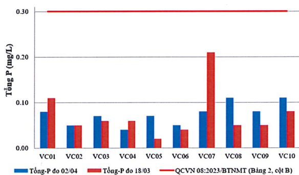
Hình 8: Biểu đồ giá trị tổng P tại các vị trí lấy mẫu ngày 01-03/04
