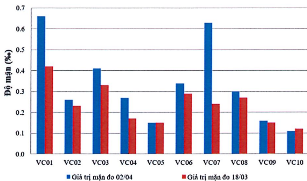
Hình 3: Biểu đồ giá trị mặn tại các vị trí lấy mẫu ngày 01-03/04
