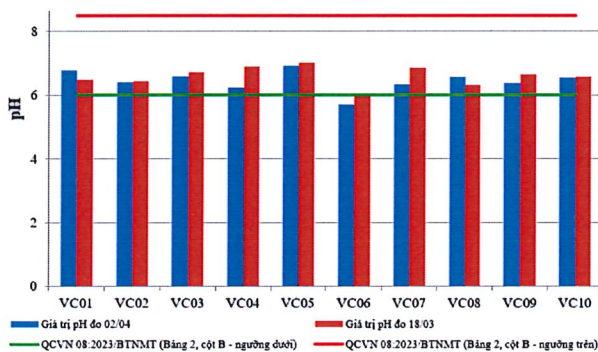
Hình 2: Biểu đồ giá trị pH tại các vị trí lấy mẫu ngày 01-03/04
