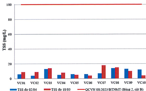
Hình 4: Biểu đồ giá trị TSS tại các vị trí lấy mẫu ngày 01-03/04
