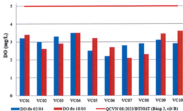
Hình 5: Biểu đồ giá trị DO tại các vị trí lấy mẫu ngày 01-03/04
