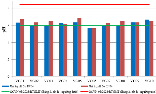
Hình 2: Biểu đồ giá trị pH tại các vị trí lấy mẫu ngày 16-18/04
