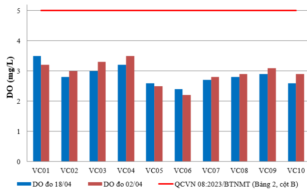
Hình 5: Biểu đồ giá trị DO tại các vị trí lấy mẫu ngày 16-18/04
