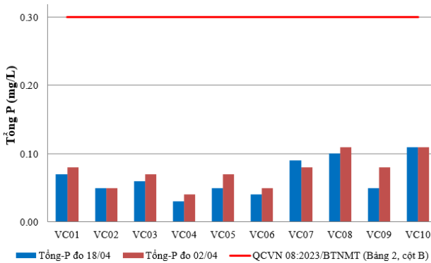
Hình 8: Biểu đồ giá trị tổng P tại các vị trí lấy mẫu ngày 16-18/04
