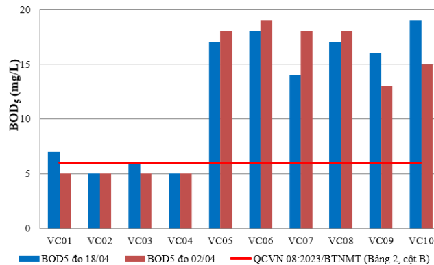
Hình 6: Biểu đồ giá trị BOD 5 tại các vị trí lấy mẫu ngày 16-18/04
