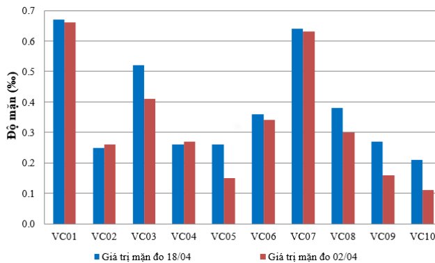
Hình 3: Biểu đồ giá trị mặn tại các vị trí lấy mẫu ngày 16-18/04
