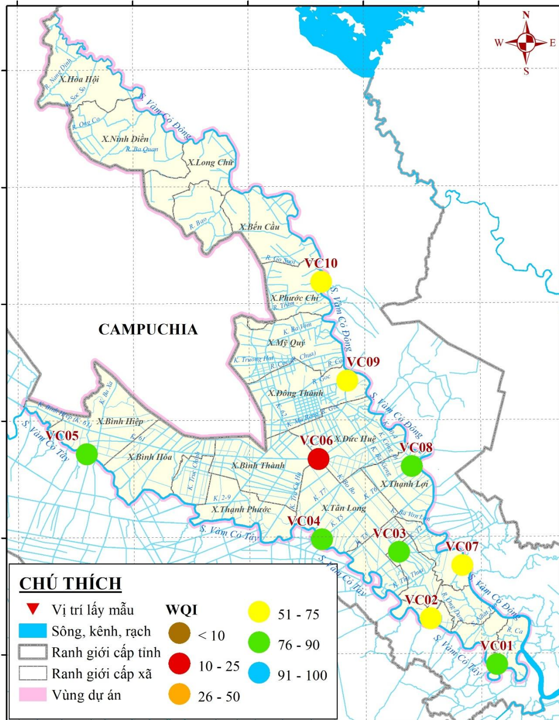
Hình 10: Biểu thị chỉ số WQI tại các vị trí lấy mẫu ngày 16-18/04/2026
