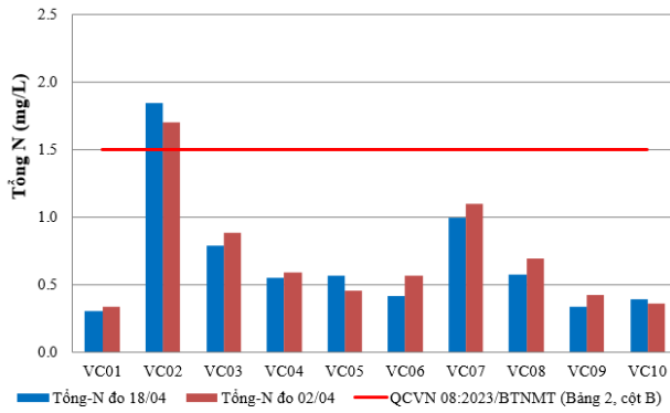
Hình 7: Biểu đồ giá trị tổng N tại các vị trí lấy mẫu ngày 16-18/04
