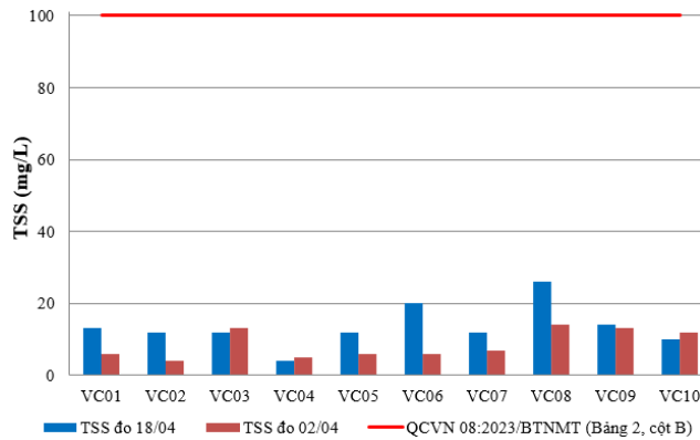
Hình 4: Biểu đồ giá trị TSS tại các vị trí lấy mẫu ngày 16-18/04
