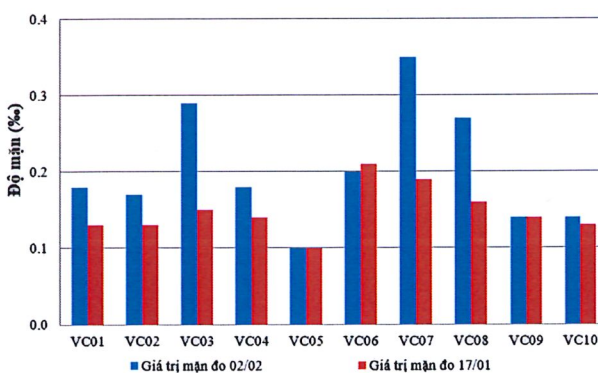
Hình 3: Biểu đồ giá trị mặn tại các vị trí lấy mẫu ngày 01-02/02
