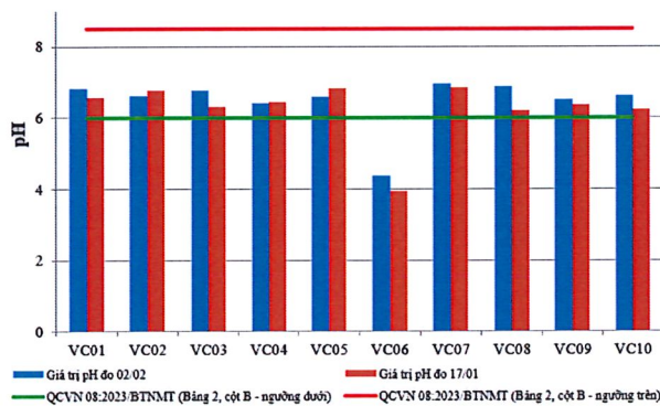
Hình 2: Biểu đồ giá trị pH tại các vị trí lấy mẫu ngày 01-02/02
