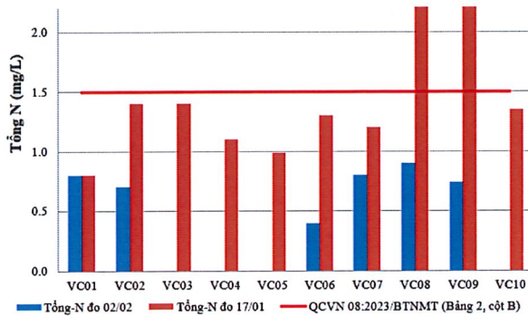
Hình 7: Biểu đồ giá trị tổng N tại các vị trí lấy mẫu ngày 01-02/02
