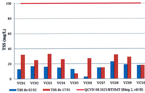
Hình 4: Biểu đồ giá trị TSS tại các vị trí lấy mẫu ngày 01-02/02
