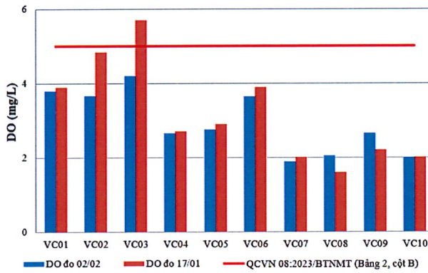
Hình 5: Biểu đồ giá trị DO tại các vị trí lấy mẫu ngày 01-02/02
