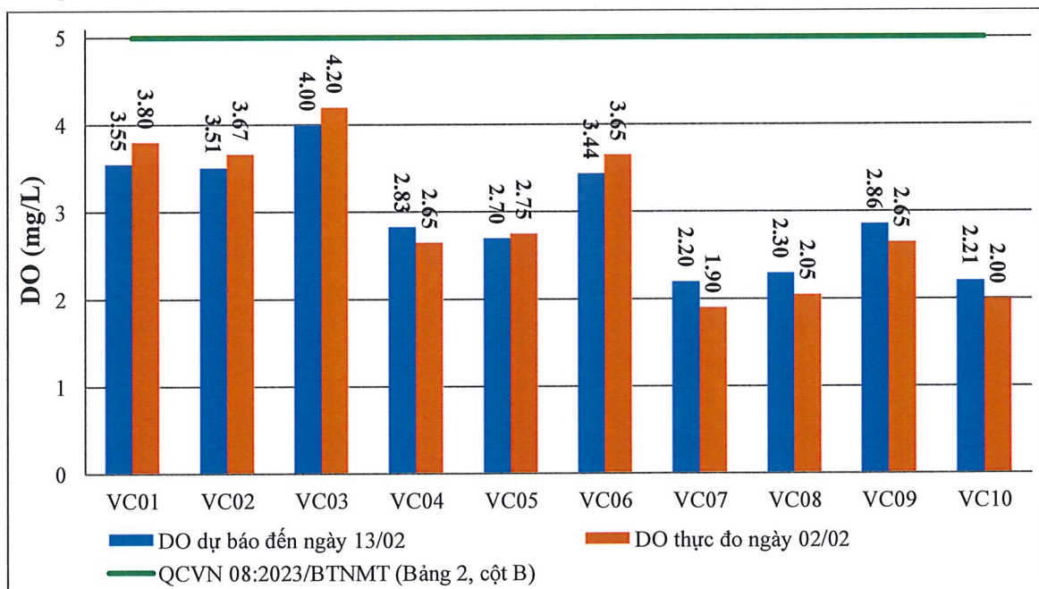
Hình 11: Biểu đồ so sánh kết quả dự báo nồng độ DO
