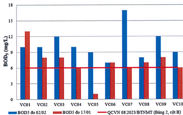
Hình 6: Biểu đồ giá trị BOD 5 tại các vị trí lấy mẫu ngày 01-02/02
