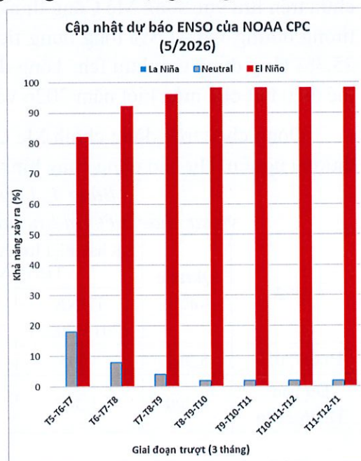
Hình 5. Dự báo diễn biến ENSO theo tháng trượt 3 tháng
